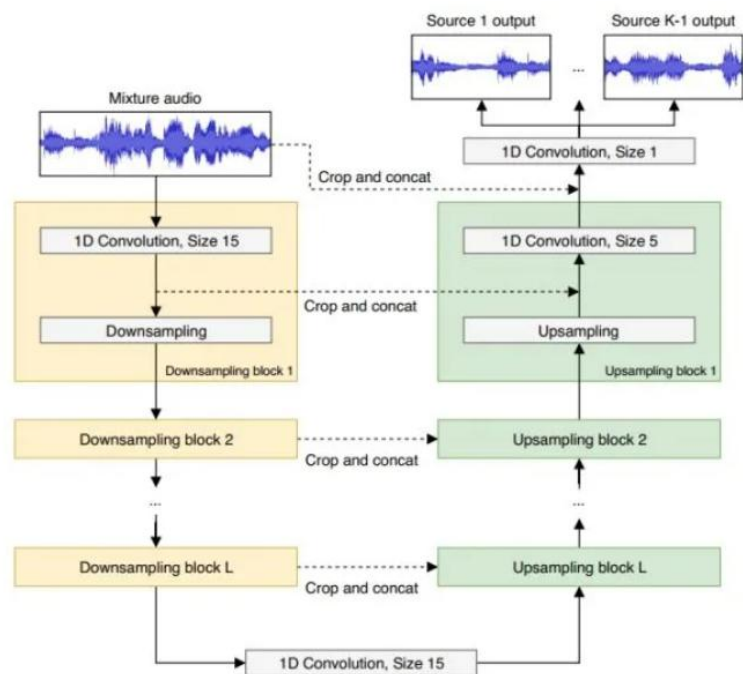
Wave-U-Net示意图
